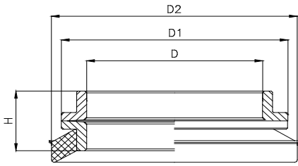
DD-KESİT
