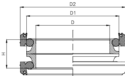
DD-KESİT
