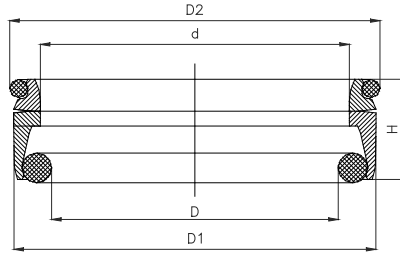
OS-KESİT
