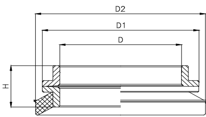
DD-KESİT
