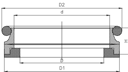
OS-KESİT
